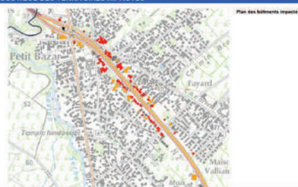
Illustration 2: Exemple de fiches voiries réalisées dans le cadre de l'étude des RN à forts enjeux
